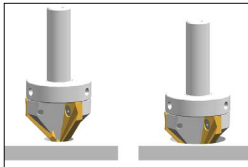
Grosser Senkbereich Large countersink range
