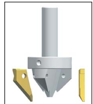
Messer auswechselbar Interchangeable blades
